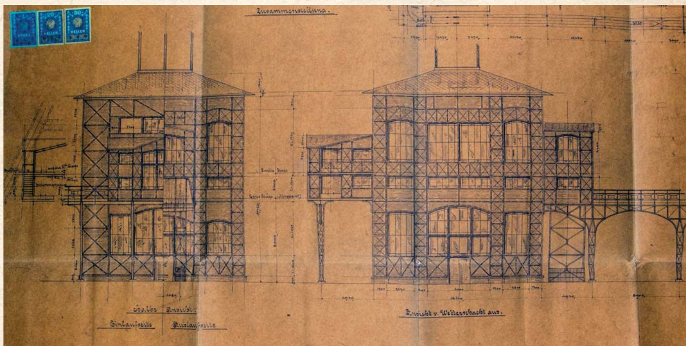
Detail stavebního plánu jámové budovy těžní věže z roku 1909. Státní okresní archiv Karviná.
