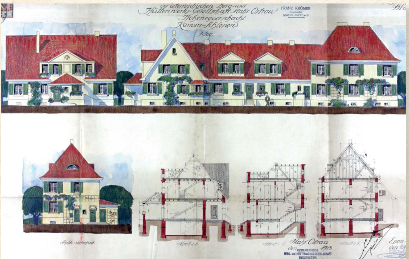
Plán domu z hornické kolonie „Nový Jork“, kterou nechala pro zaměstnance dolů Hohenegger a Austria (Barbora) nechala v Karviné postavit v letech 1913-1917 Rakouská báňská a hutní společnost. Jednalo se o první kolonii v Ostravsko-karvinském revíru, kde byly využity principy zahradního města. Státní okresní archiv Karviné.
