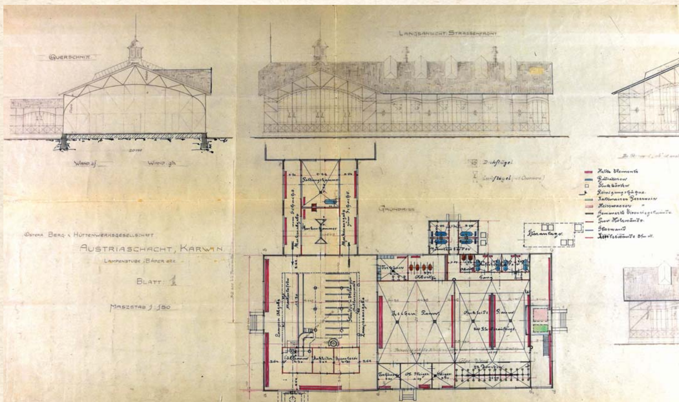
Stavební plány lampovny a koupelen z roku 1910. Státní okresní archiv Karviná.
