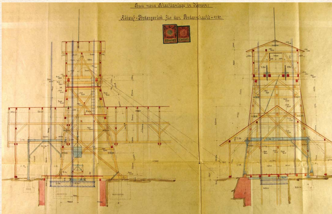
Výřez stavebního plánu hloubičího zařízení těžní jámy z roku 1907. Státní okresní archiv Karviná.
